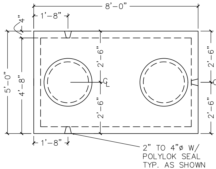
TOP VIEW N.T.S.
