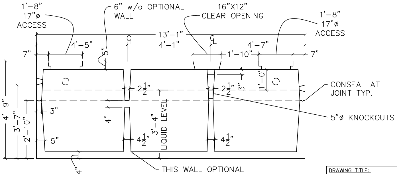
TOP VIEW N.T.S.
